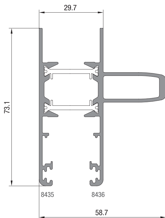
RPT-032 1.500 kg/m
