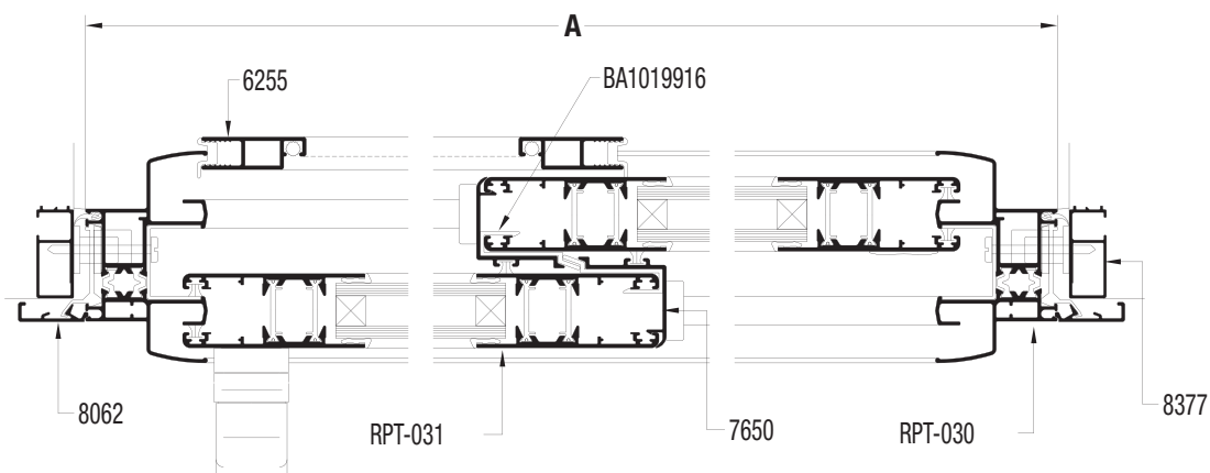
SECCIÓN 1-2-3
