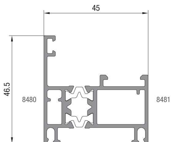
RPT-035 1.032 kg/m
