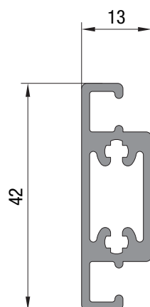
6256 0.543 kg/m
