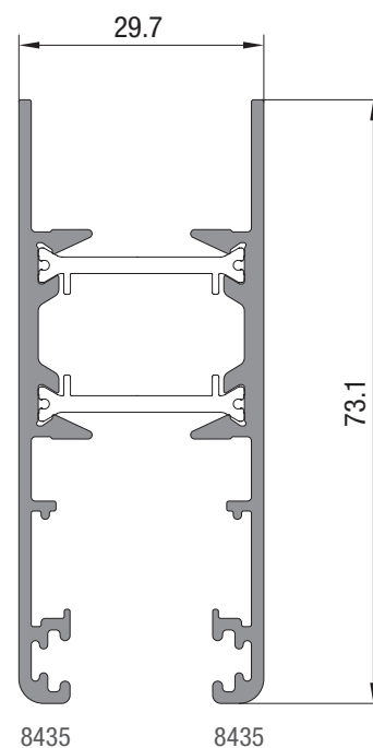
RPT-031 1.192 kg/m
