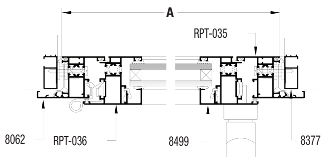
SECCIÓN 1-2
