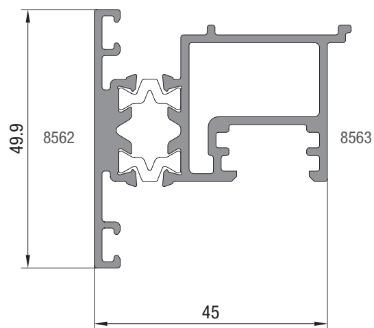
RPT-047 1.240 kg/m
