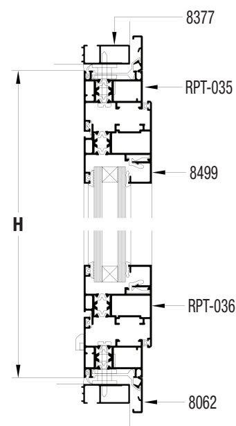
SECCIÓN 3-4
